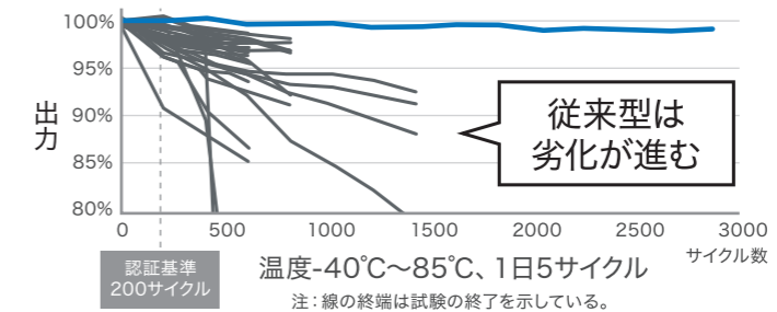
温度サイクル試験
