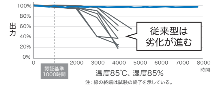
高温多湿試験
